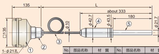
垂直取付での上限検出用 L寸法Max6000mm
